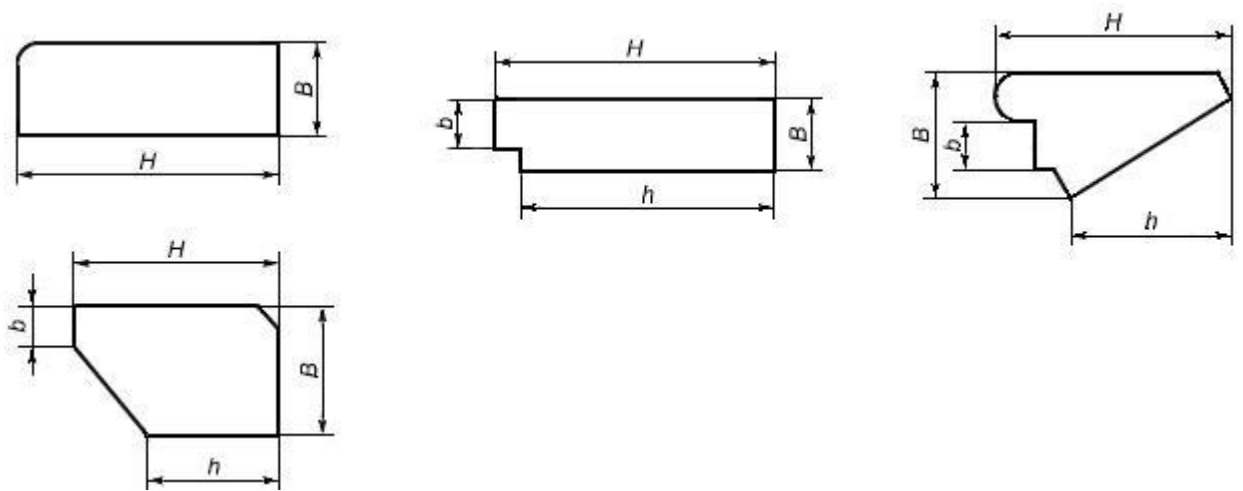
Рисунок 5 - Целые ступени
