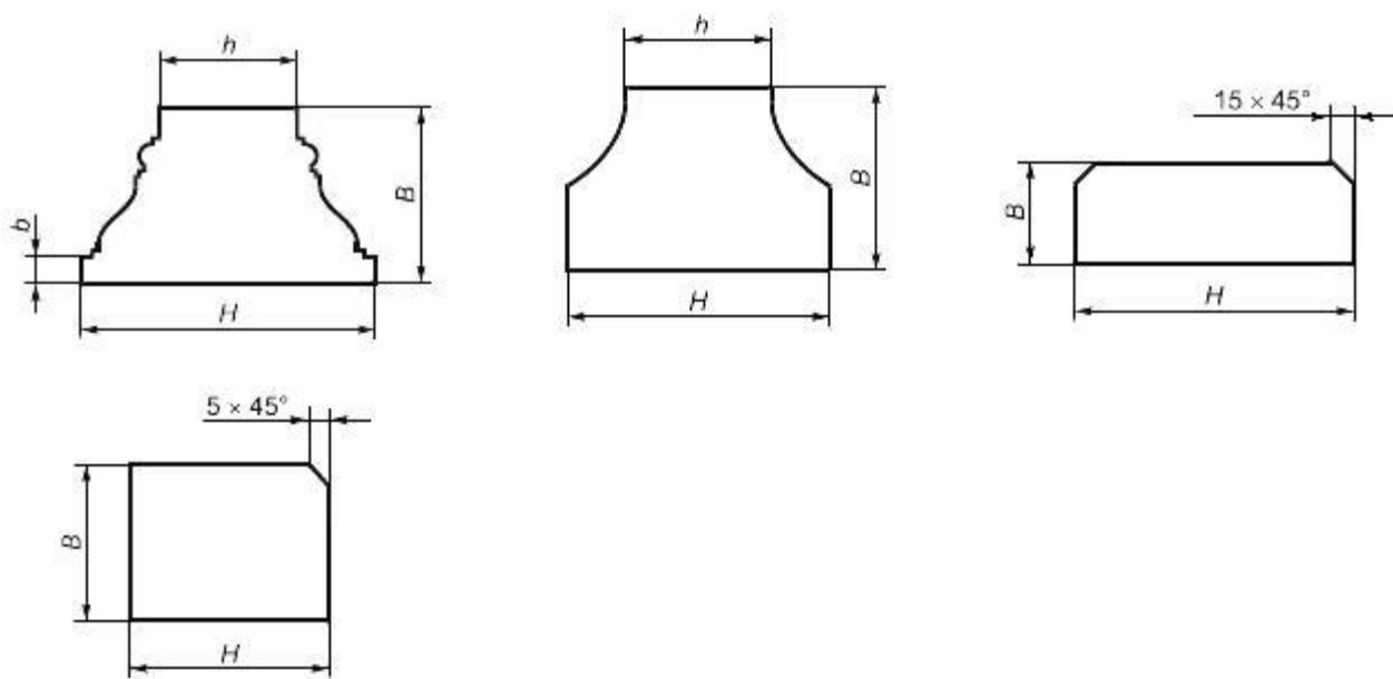
Рисунок 8 - Основания балюстрад
