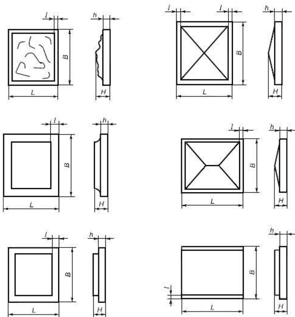
Рисунок 1 - Рустовые камни
