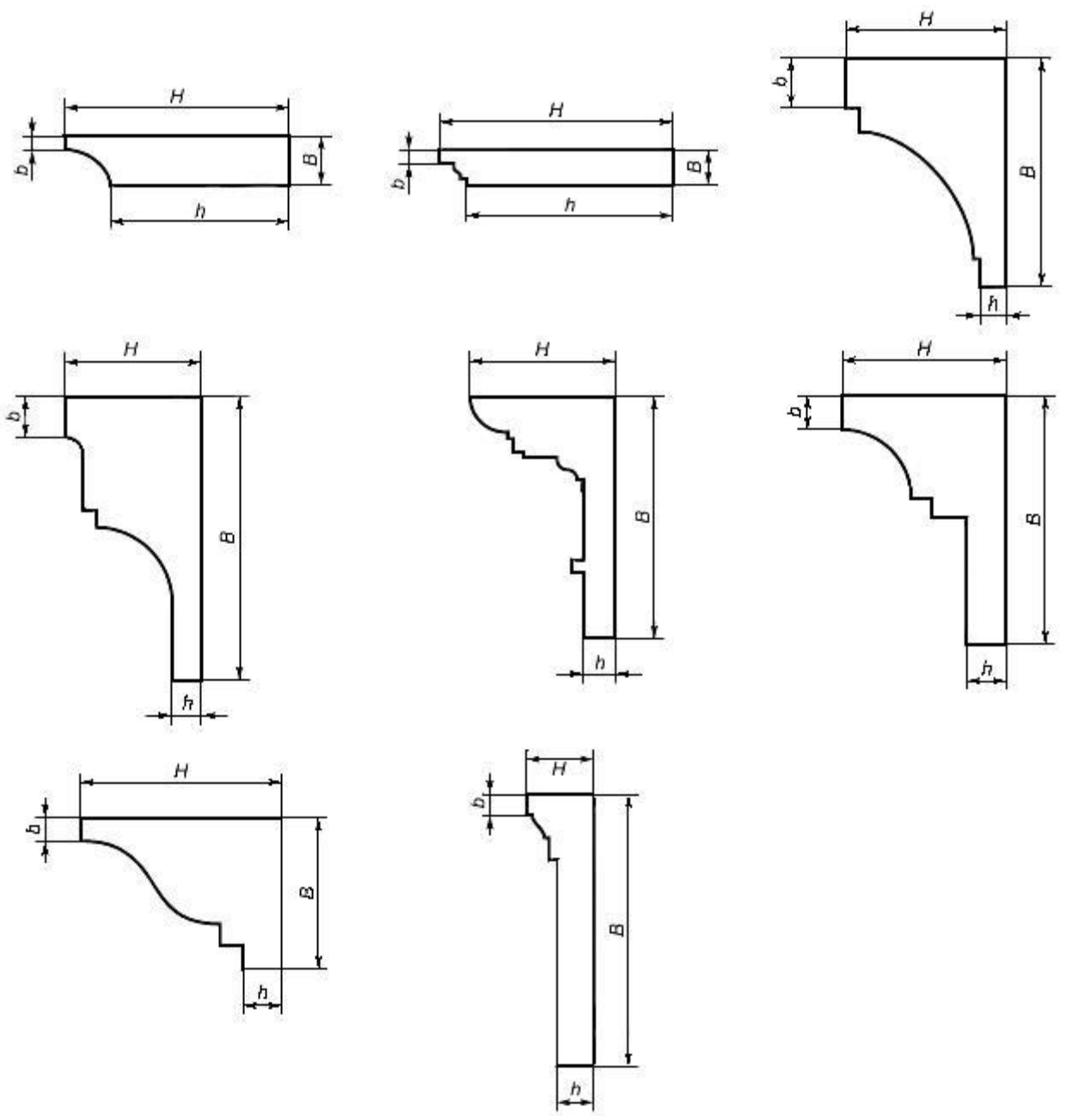
Рисунок 3 - Карнизы
