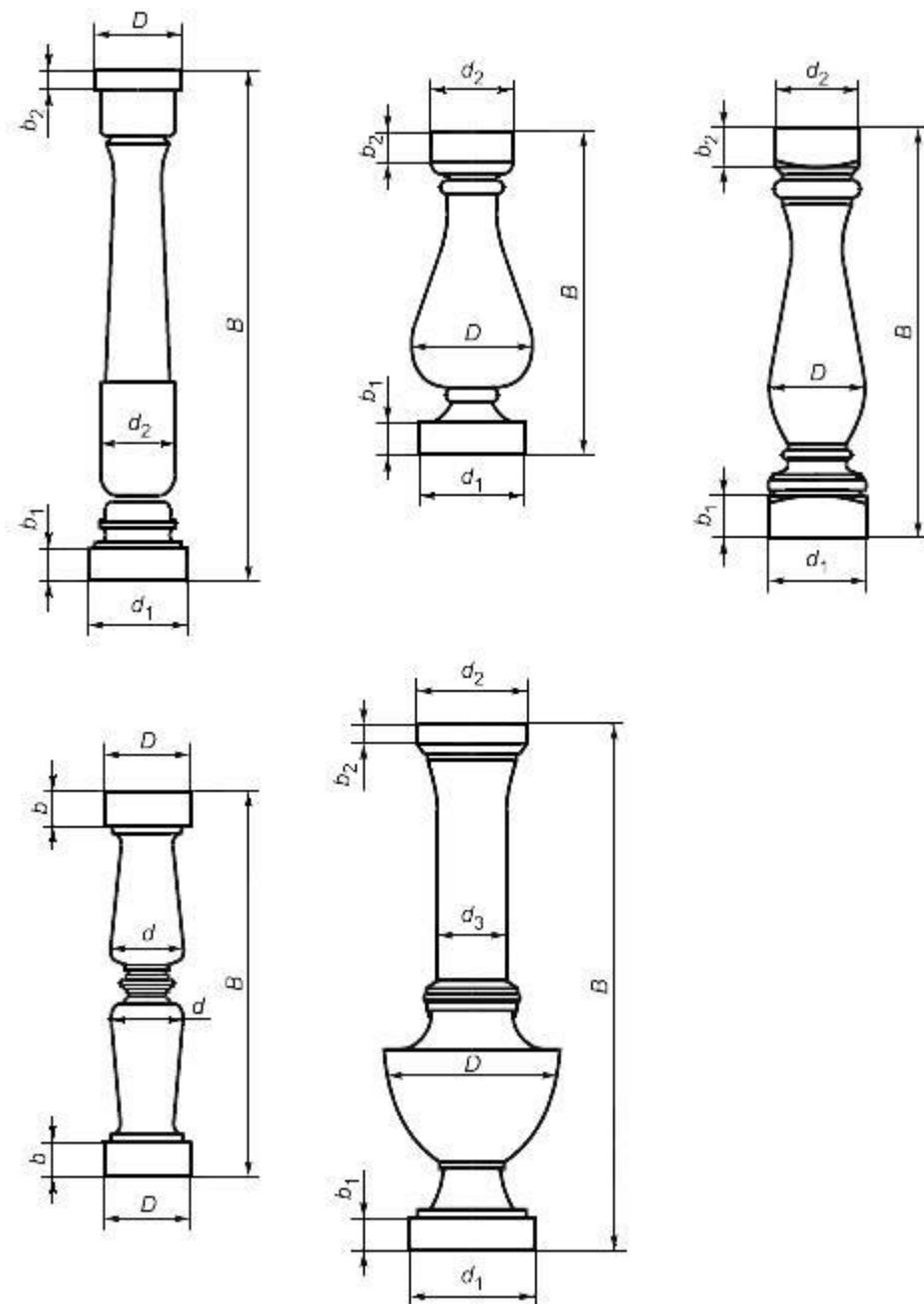
Рисунок 11 - Балюсины
