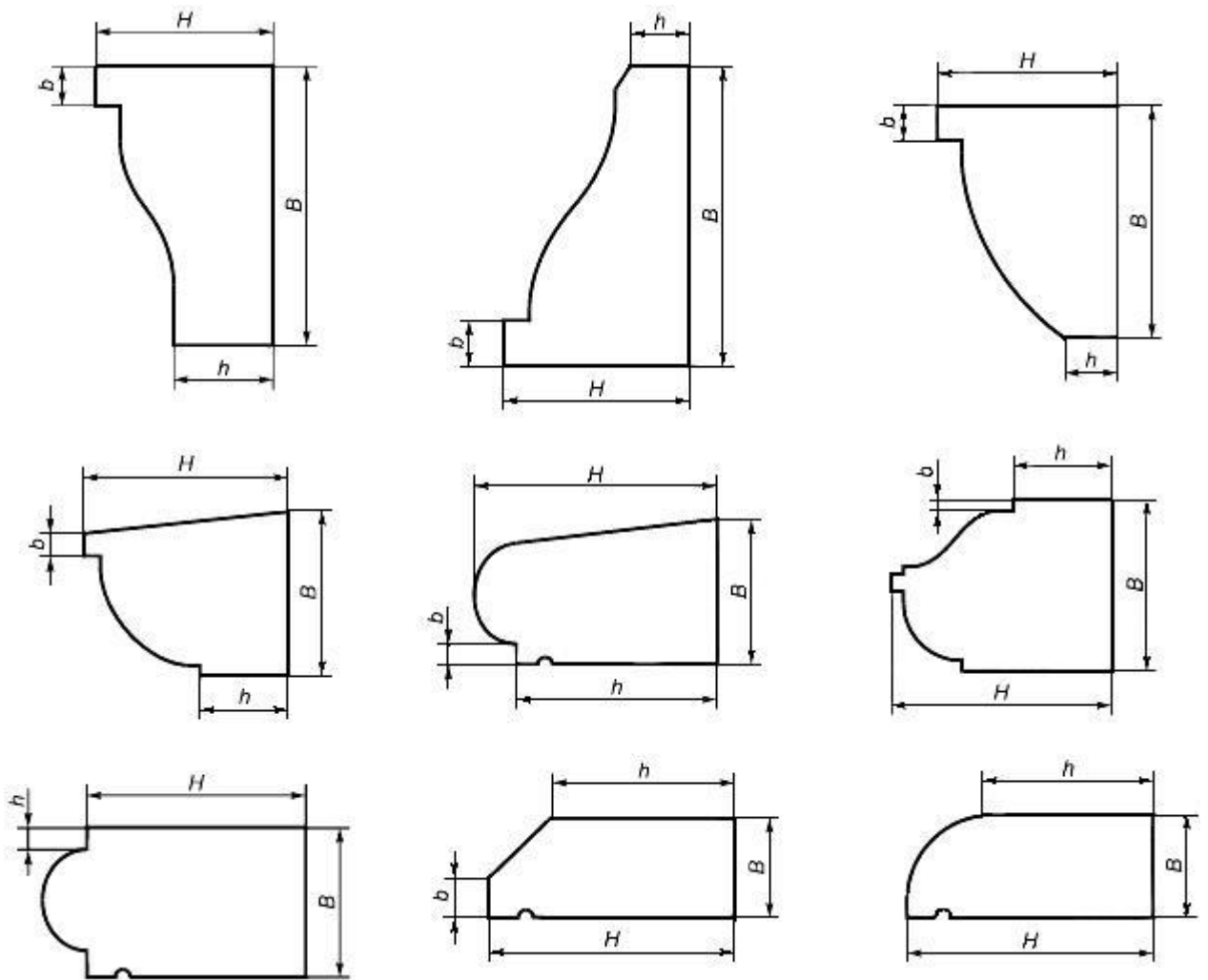
Рисунок 4 - Кордонные камни
